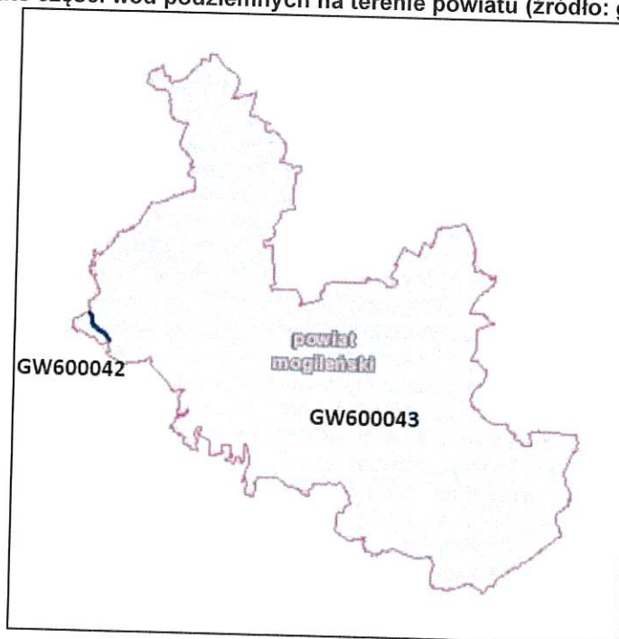
Rysunek 4 Jednolite części wód podziemnych na terenie powiatu (źródło: geoportal.gov.pl)
